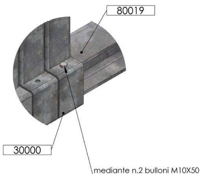
Figura 14: Dettaglio bulloni sacrificali binari
