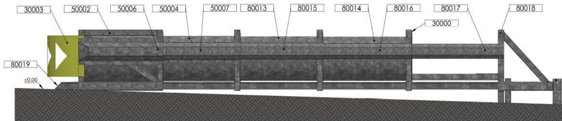
Figura 17: Attenuatore ZMP80 (vista laterale)
