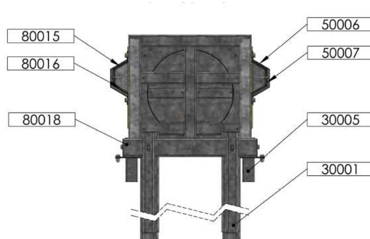
Figura 18: Attenuatore ZMP80 (vista frontale e posteriore)
