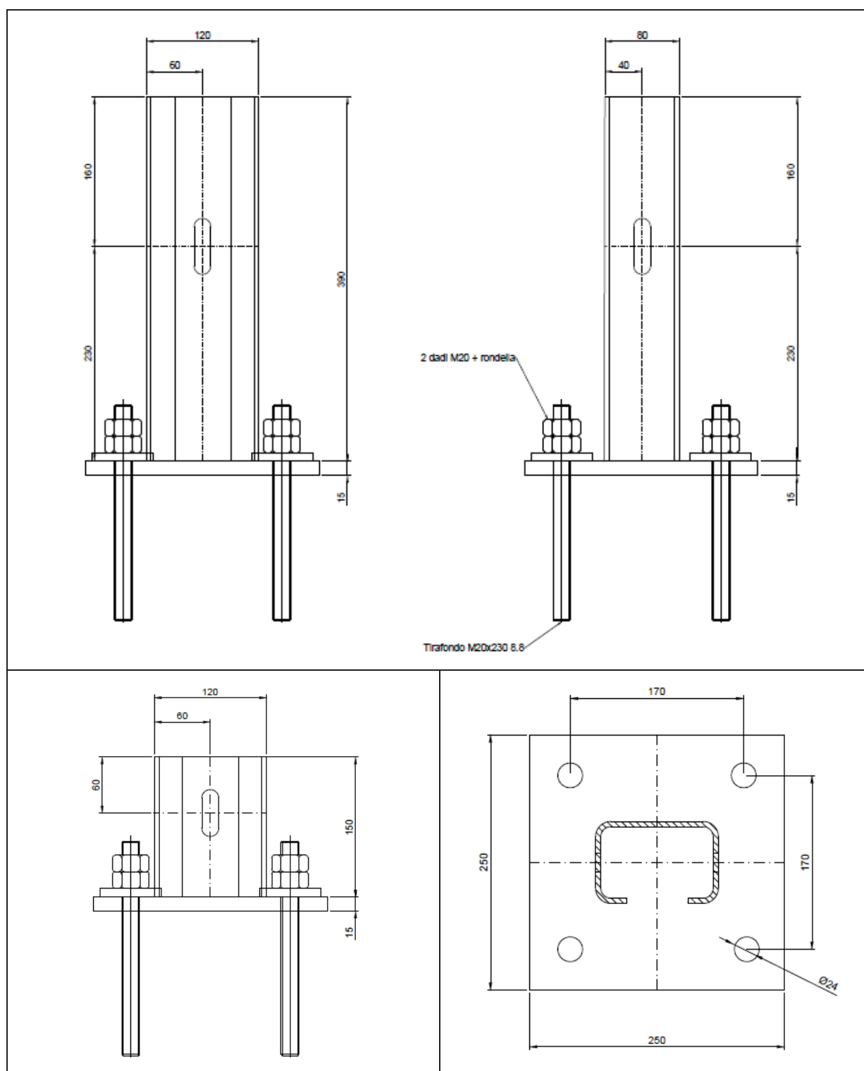
Figura 12: Paletti speciali per installazione su calcestruzzo
