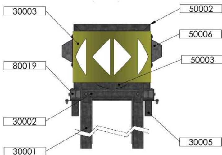
Figura 18: Attenuatore ZMP80 (vista frontale e posteriore)
