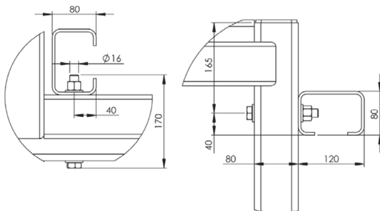
Figura 8: Dettaglio E ed F
