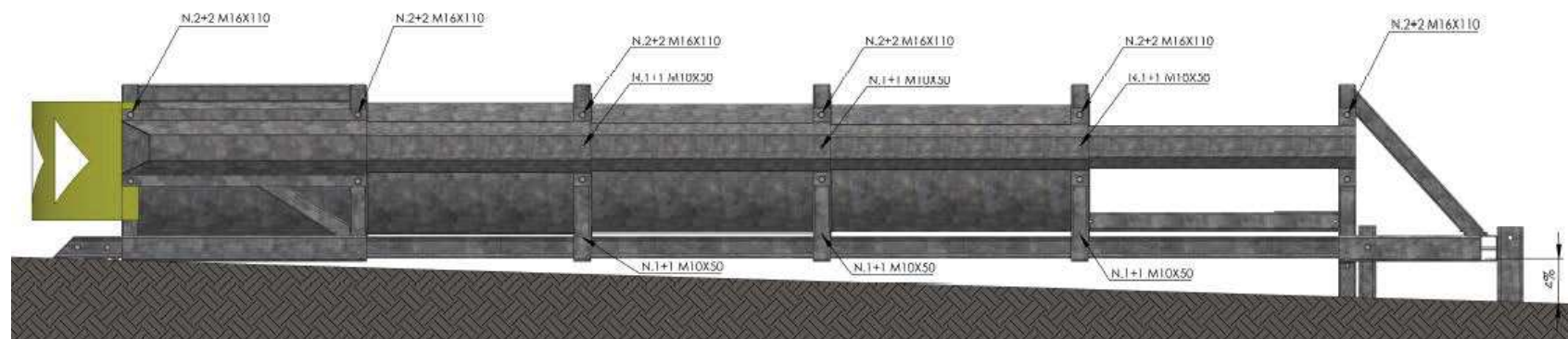
Figura 19: indicazione bulloneria ZMP80
